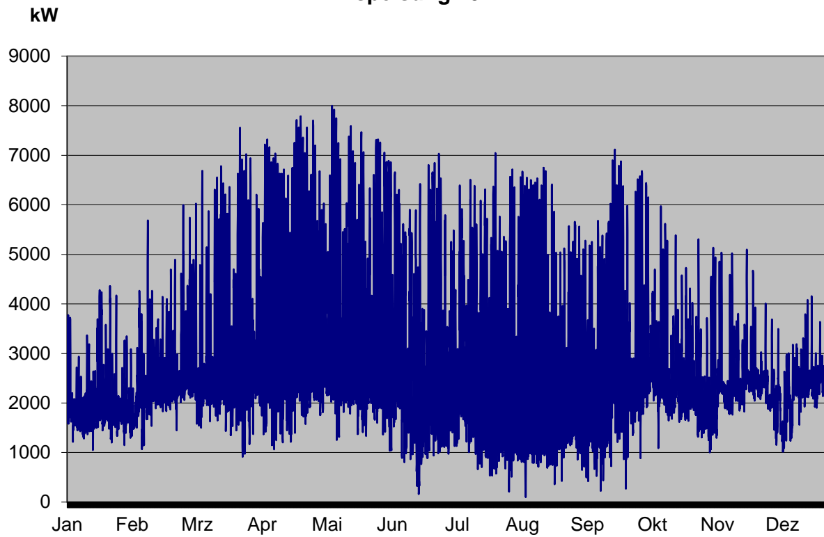
Einspeisung 20 kV
