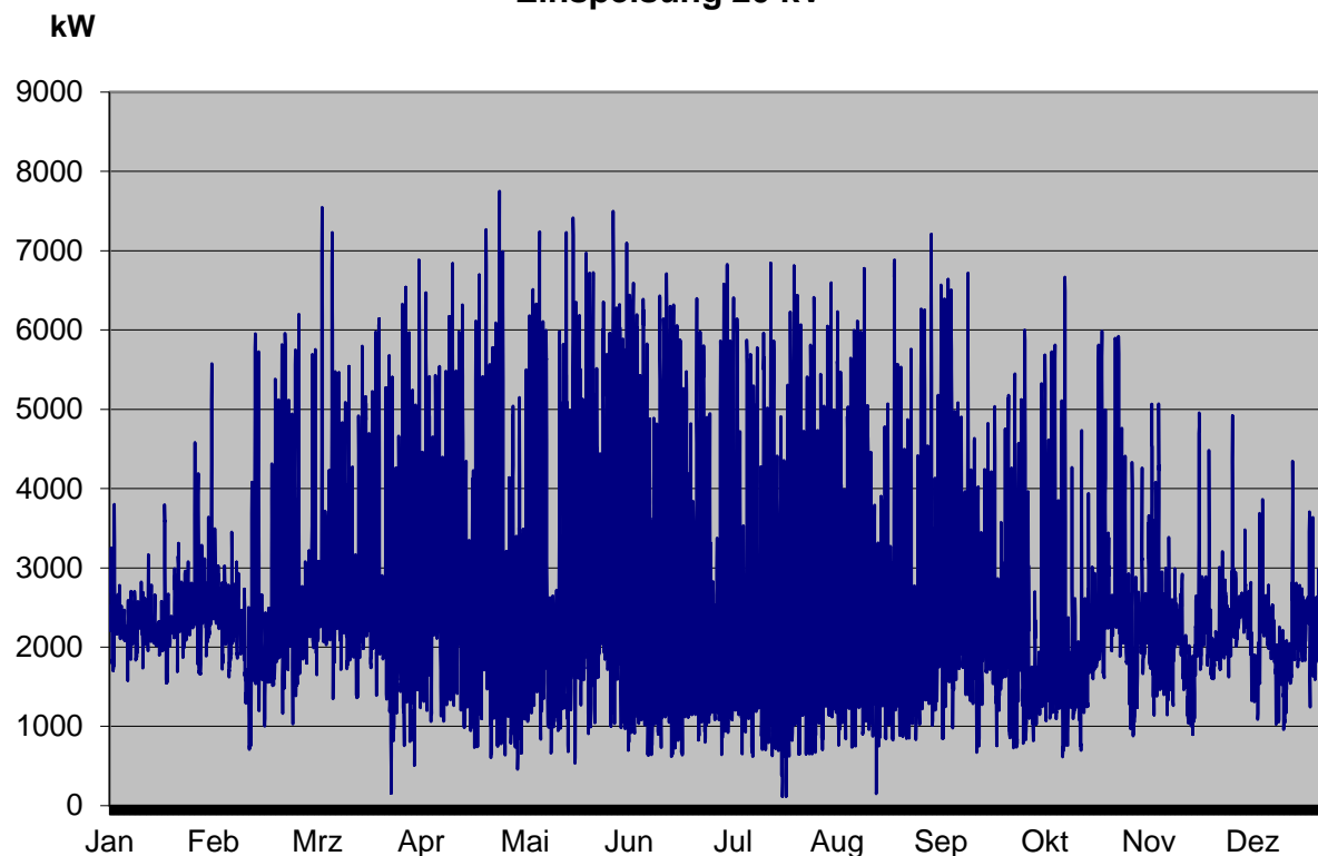
Einspeisung 20 kV
