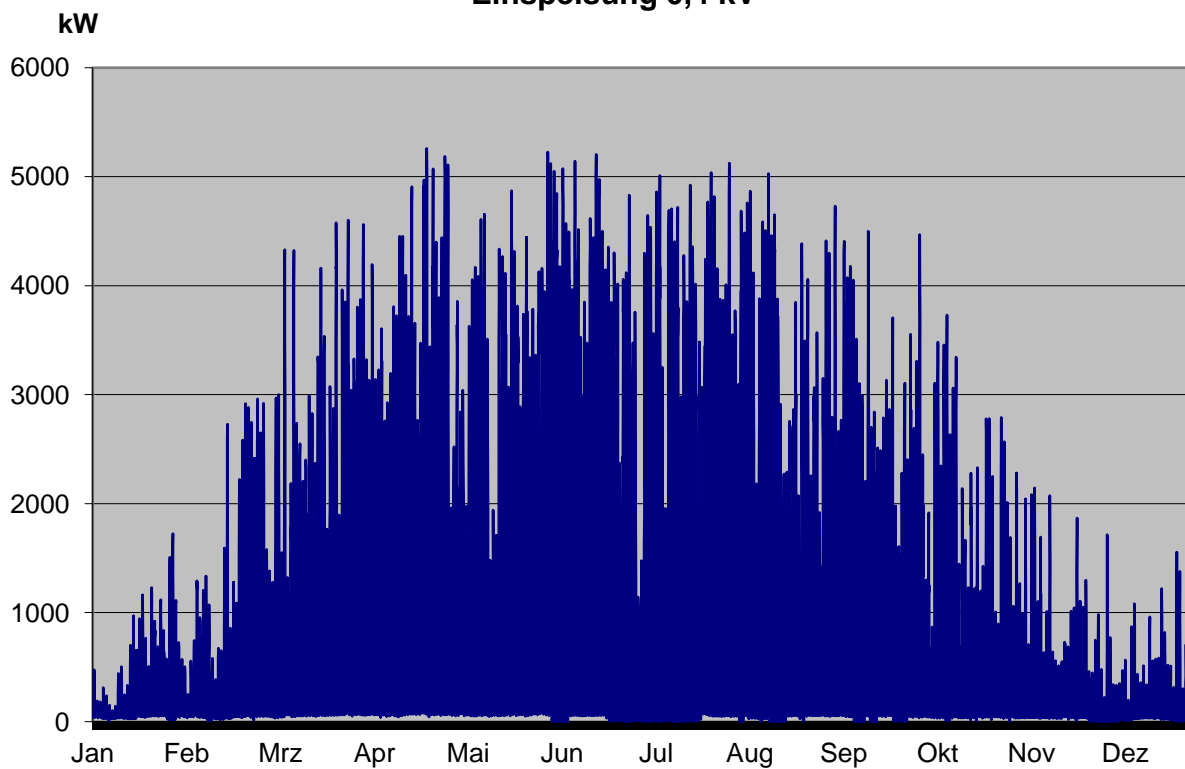
Einspeisung 0,4 kV
