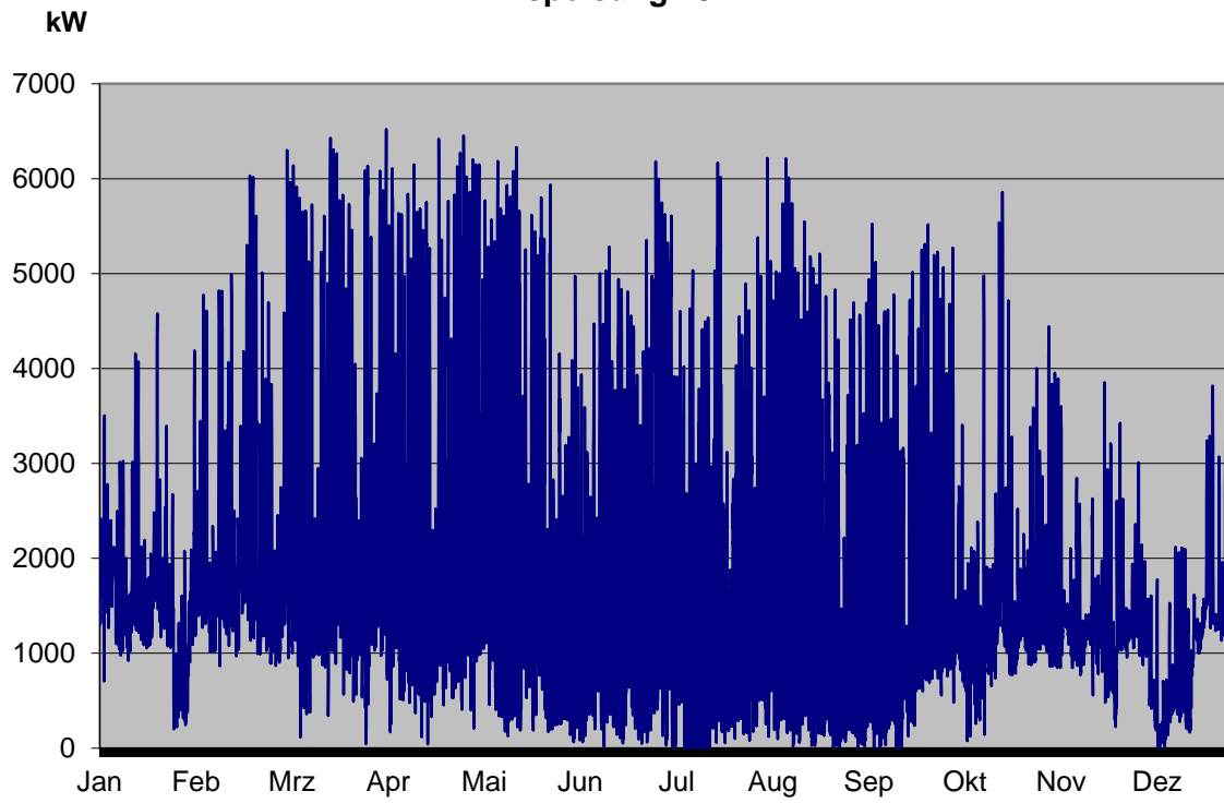
Einspeisung 20 kV
